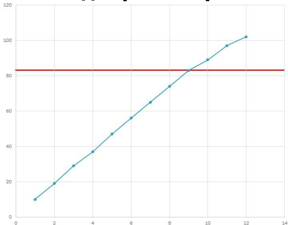
Диаграмма Парето
